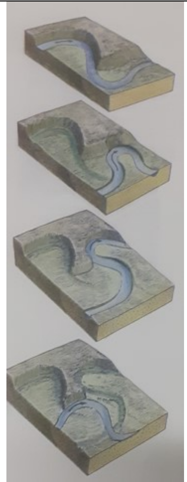
Schema della formazione di un peduncolo ad opera di un corso d'acqua meandreggiante in tempi successivi 24
